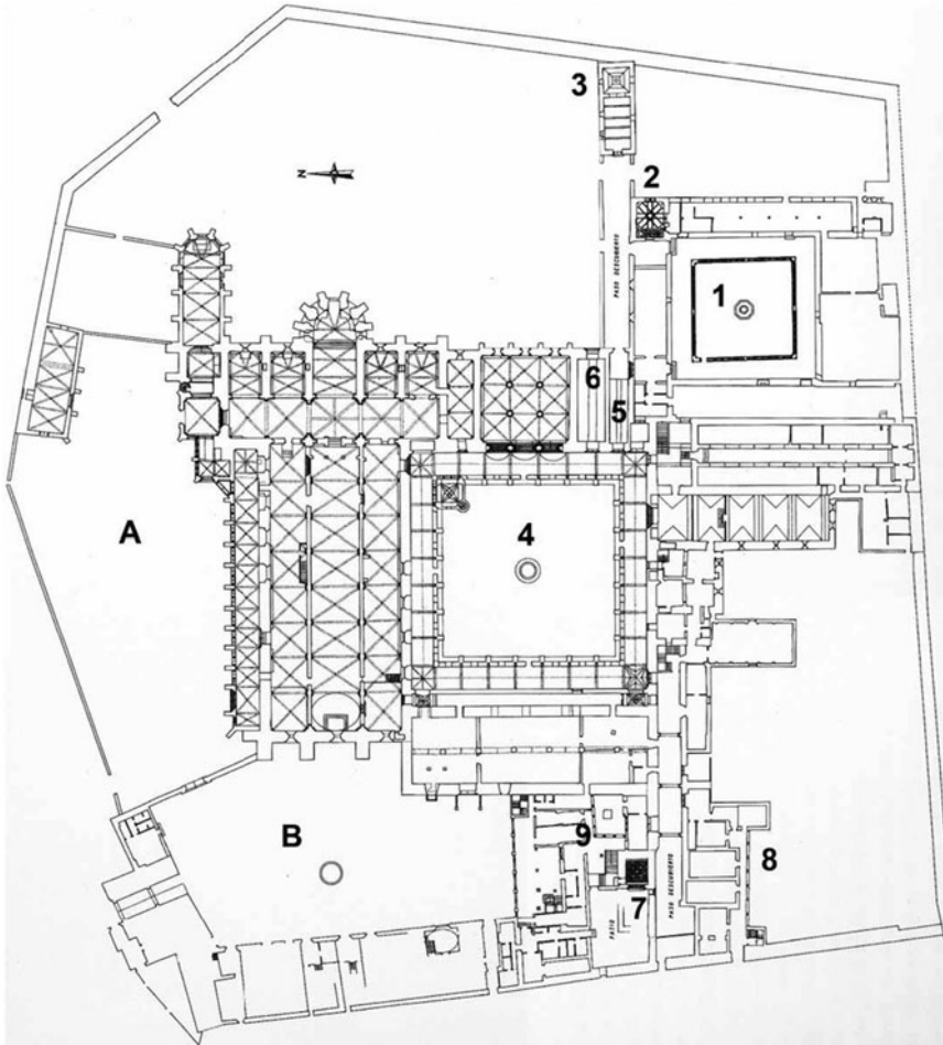
Figure 1. Santa María la Real de Las Huelgas, Burgos, ground plan. 1. Claustro de San Fernando; 2. Capilla de la Asunción; 3. Capilla de Santiago; 4. Claustro de San Fernando; 5. Pasaje (passageway); 6. Locutorio (parlour). (Adapted from Isidro Gonzalo Bango Torviso, Monjes y monasterios: El Cister en el medioevo de Castilla y León [Valladolid, 1998], 183.)
